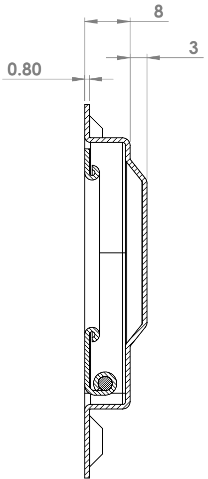
SECTION A-A SCALE 1.5 : 1
